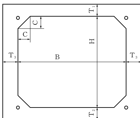
断面図
