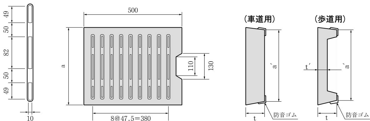
排水孔詳細図
