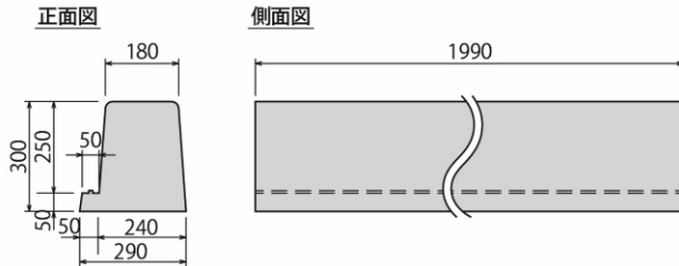
歩車道境界ブロック：両面R片防草 C
