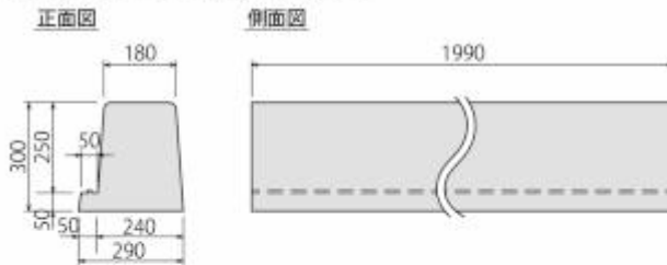
歩車道境界ブロック：両面R片防草 C
