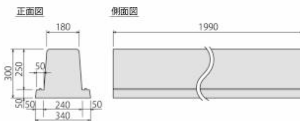
歩車道境界ブロック：両面R両防草 C
